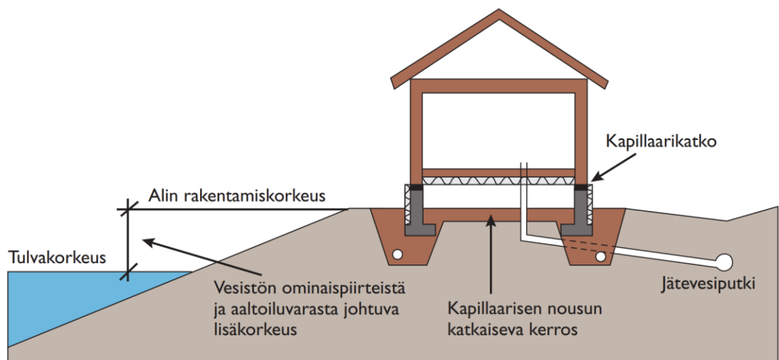
Kuva 2 Alin suositeltava rakentamiskorkeus tuulettuvalle alapohjalle. Lähde Ympäristöopas 2014
