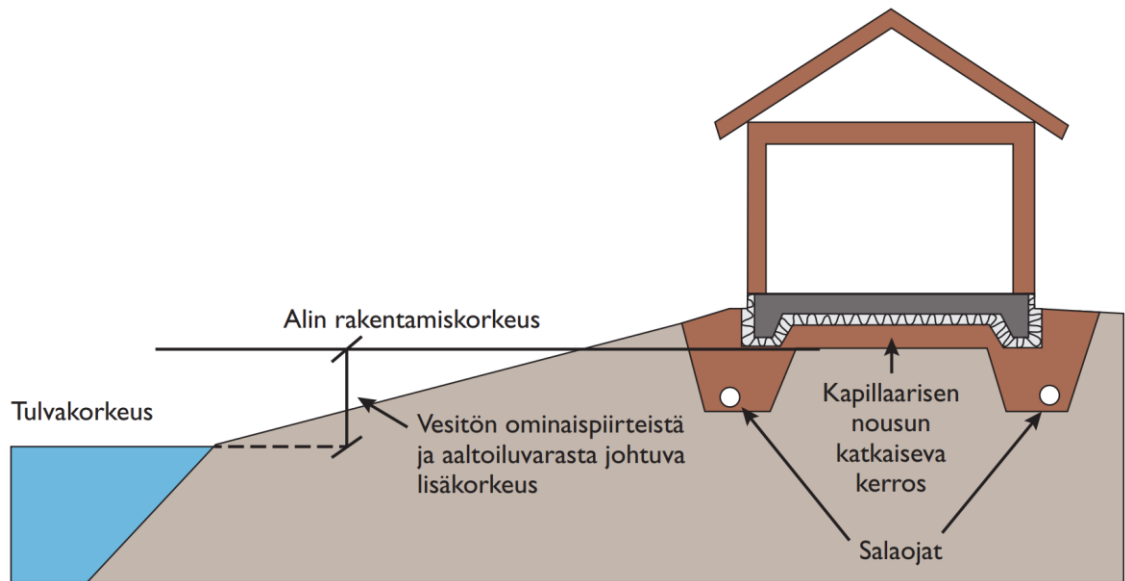
Kuva 1 Alin suositeltava rakentamiskorkeus matalaperustuksella. Lähde Ympäristöopas 2014.
